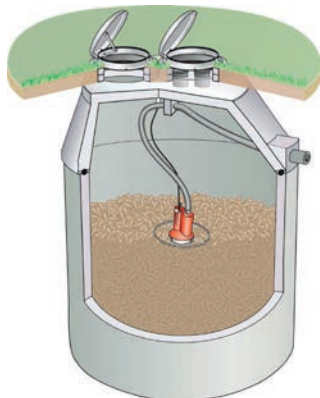
Abb. 9: Erdlager aus Beton mit Saugentnahme von oben
