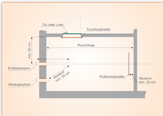
Abb. 18: Grundriss eines Pelletlagerraums
